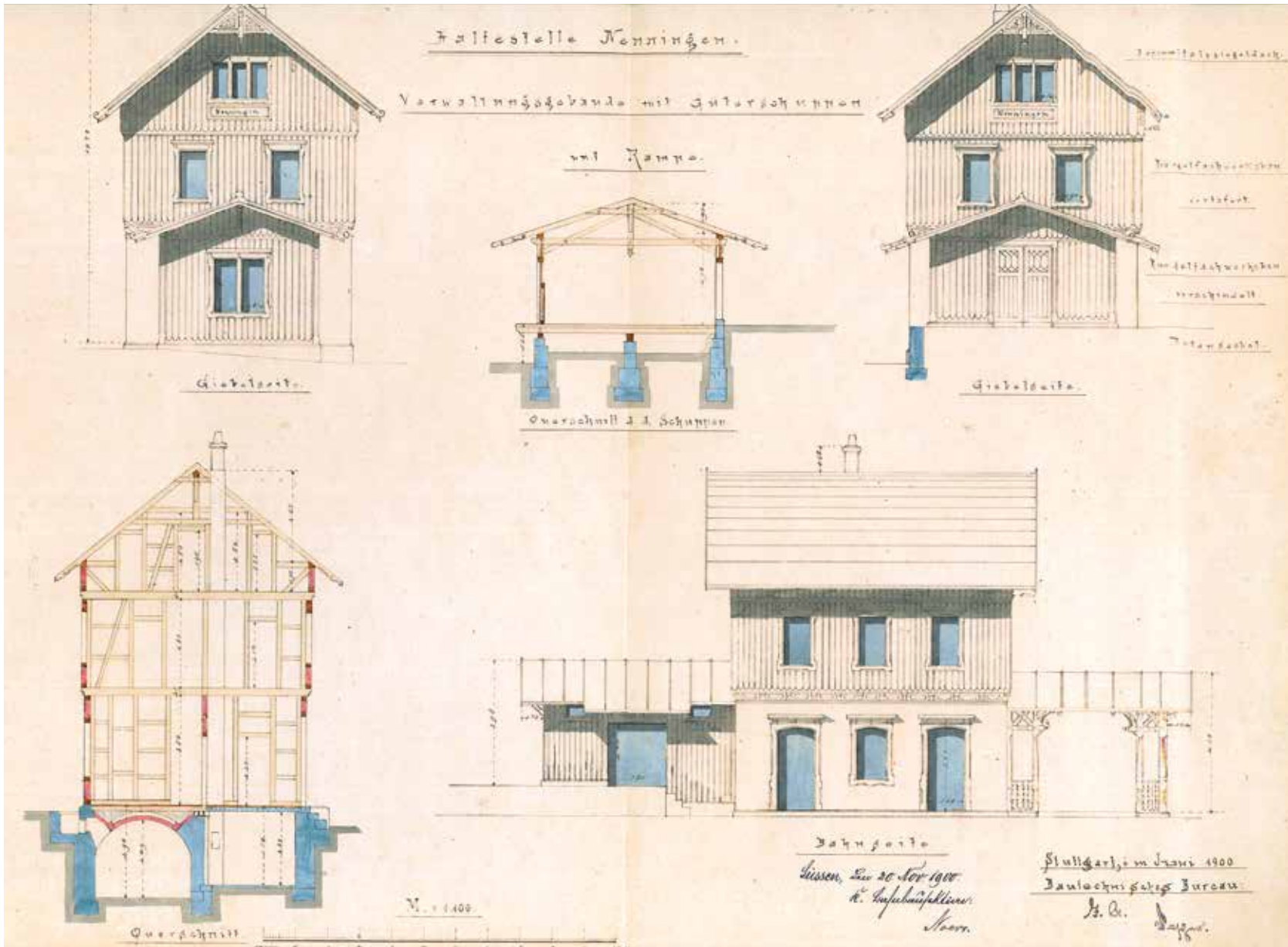
Bauplan von 1900
